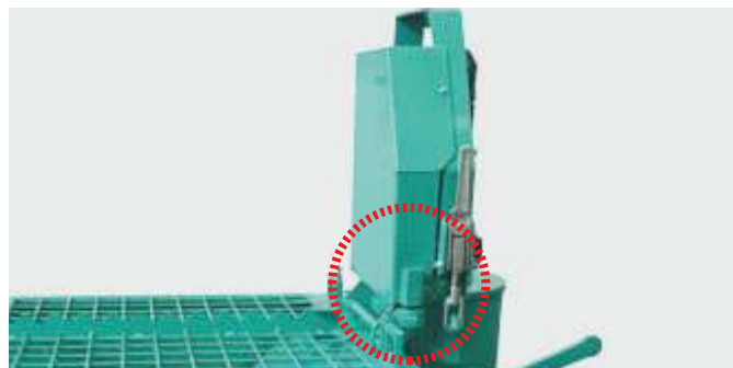
Senzor de siguranță pentru deschiderea camerei de amestecare.
